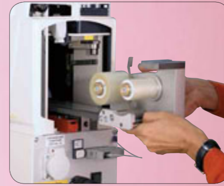
Systém aut. čištění tamponu (integrováný do stroje)
